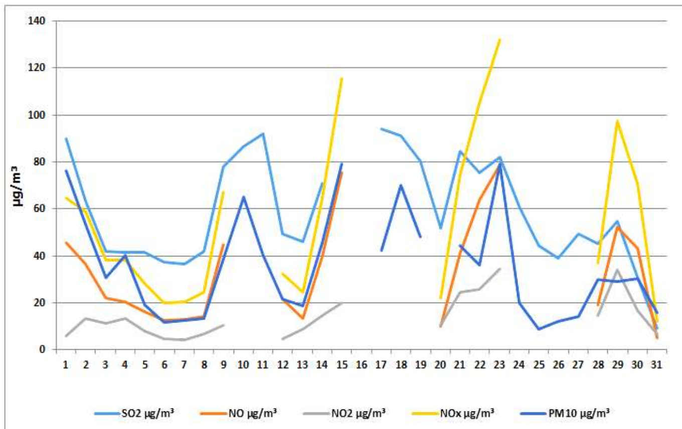
Дијаграм 5. Графички приказ просјечних имисијских дневних концентрација \text{SO}_2 , \text{PM}_{10} , \text{NO} , \text{NO}_2 и \text{NOx} за децембар 2025. у Гацку (мјерном мјесту круг ОШ „Свети Сава“).
